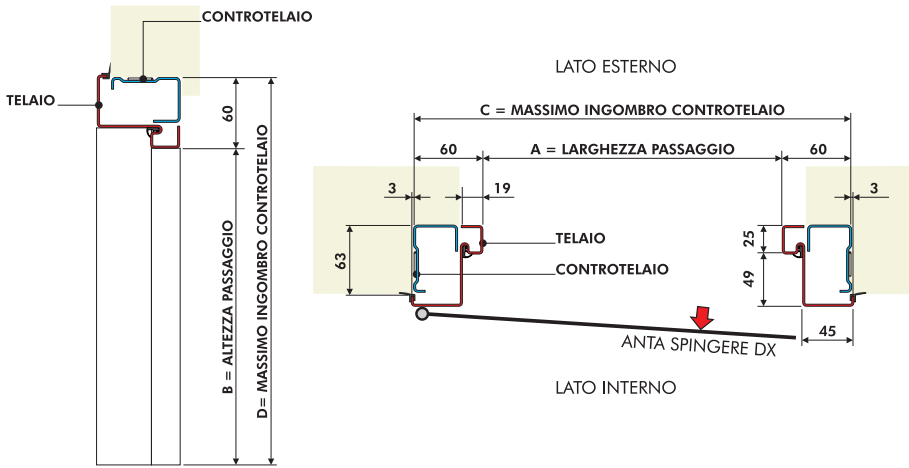
MISURE STANDARD PER IL TELAIO E CONTROTELAIO
